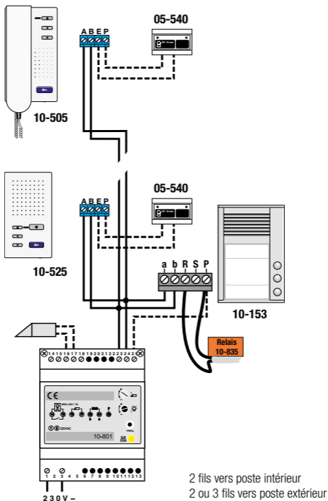
fig.1: schéma de raccordement complet
