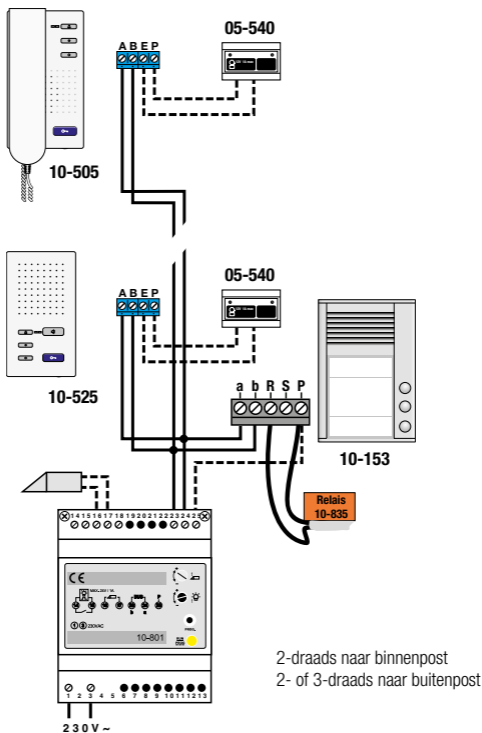
fig.1: compleet aansluitschema
