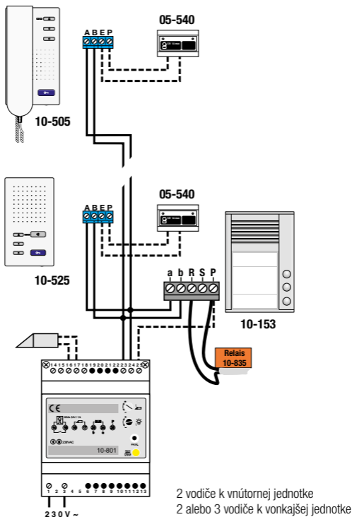
Obr. 1 Úplná schéma zapojenia
