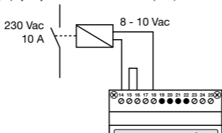
Obr. 3: Pripojenie svetelného obvodu (230V~) na NAPÁJACÍ ZDROJ 20
