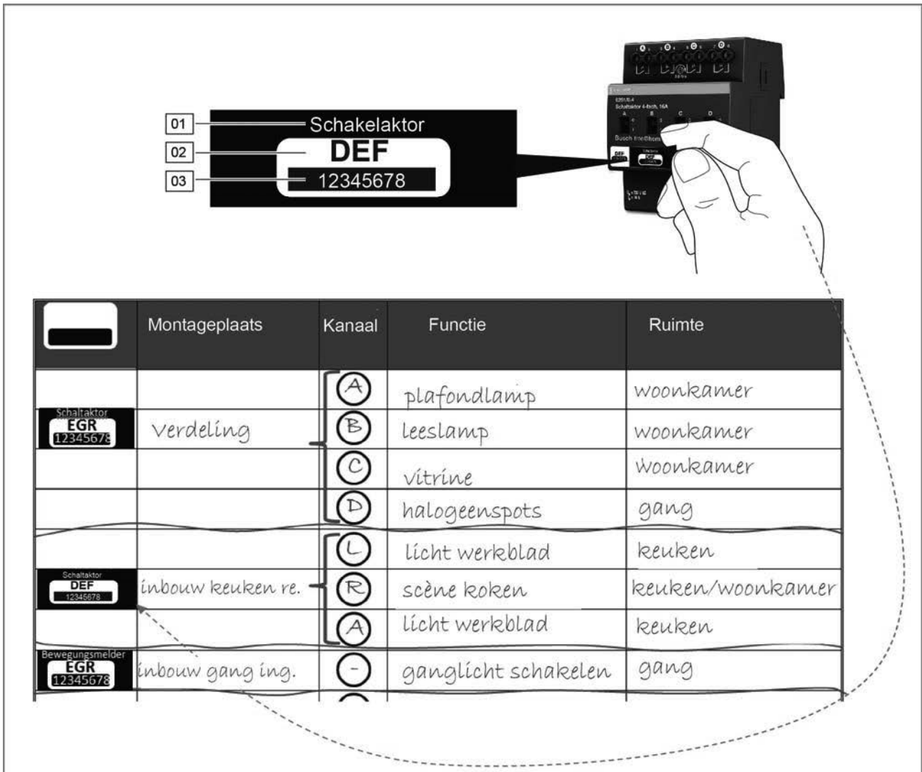
Afb. 8 Componentenschema
