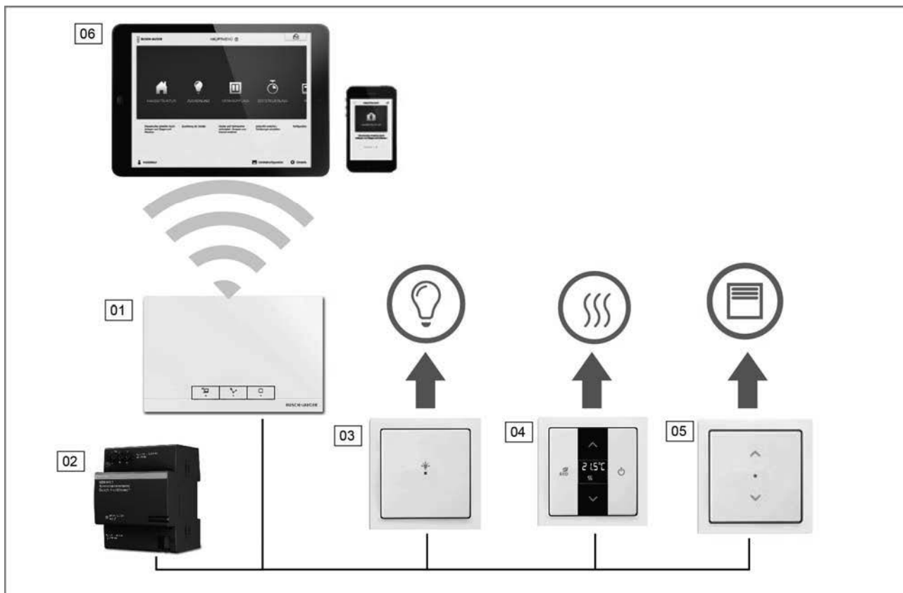
Afb. 1 Installatieplanning
