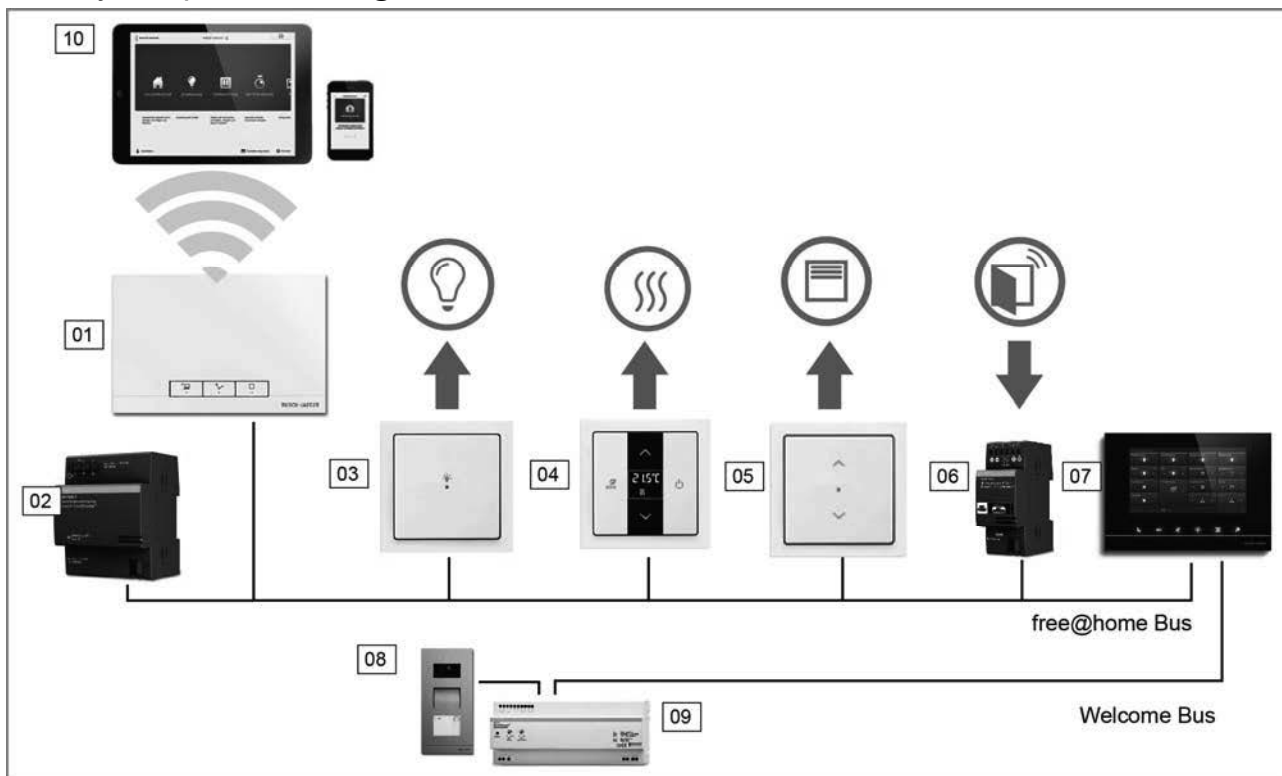
Afb. 39 Systemopbouw Busch-free@home met Busch-Welcome
