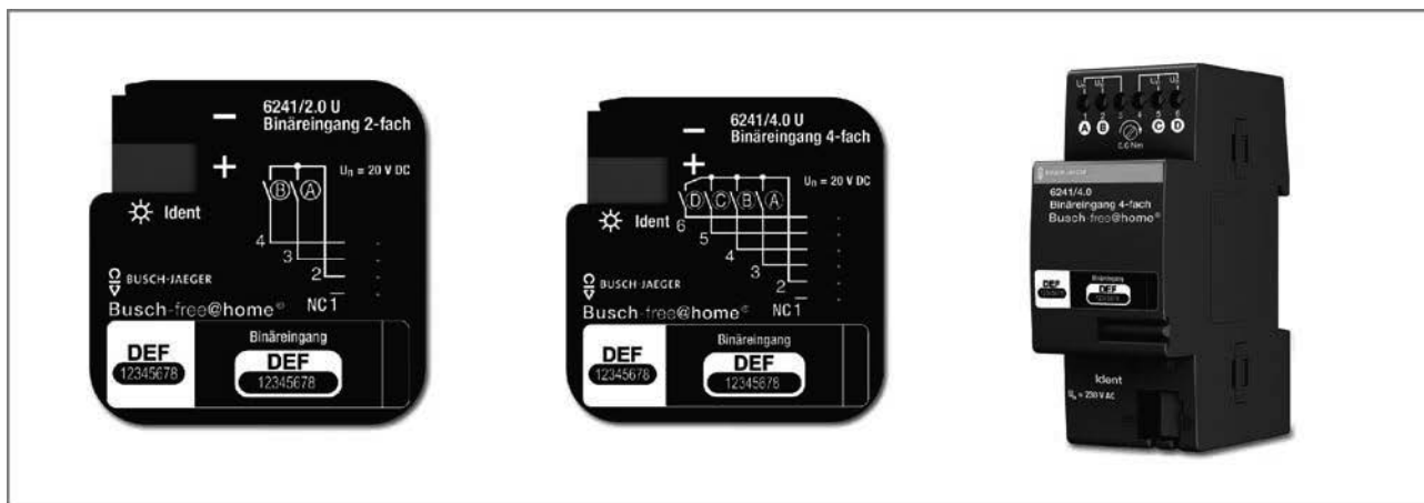
Afb. 40 Binaire ingangen
