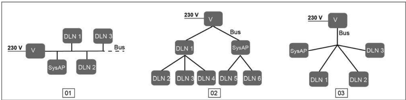
Afb. 3 Mogelijke topologieën
