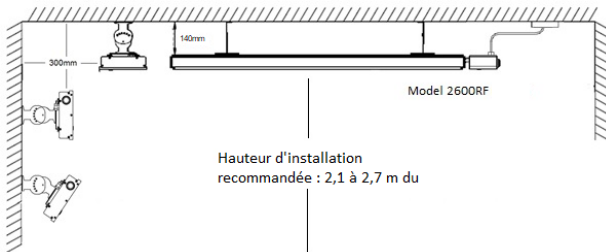
Diagramme 2 : Options de montage et distances minimales aux objets.
