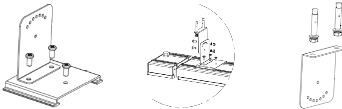
Diagramma 1: Montaggio della staffa girevole
