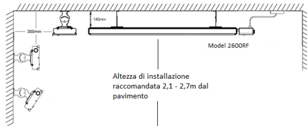
Diagramma 2: Opzioni di montaggio e distanze minime dagli oggetti.
