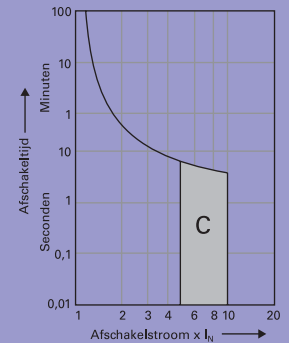
Afschakelkarakteristiek C
