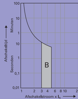
Afschakelkarakteristiek B
